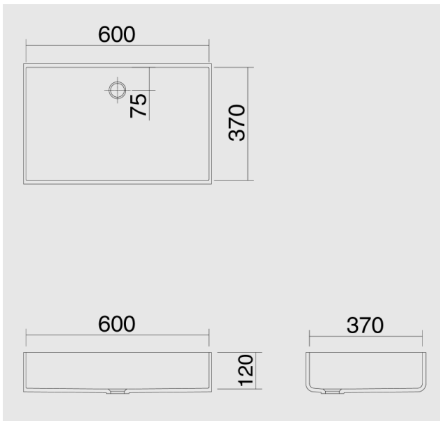
FONTANA FP-60
