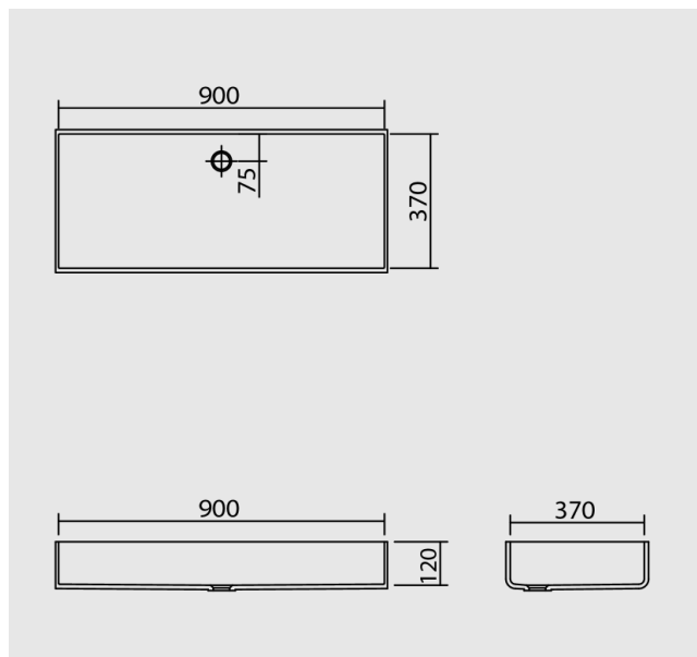
FONTANA FP-60-900
