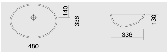
FONTANA FO-48 480 x 336 x 130 mm
