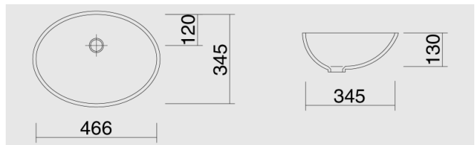
FONTANA FO-47 466 x 345 x 130 mm
