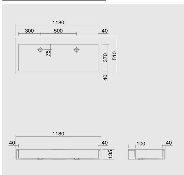
FONTANA ASP-118
