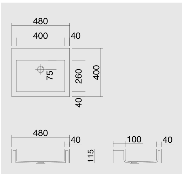
FONTANA ASP-48
