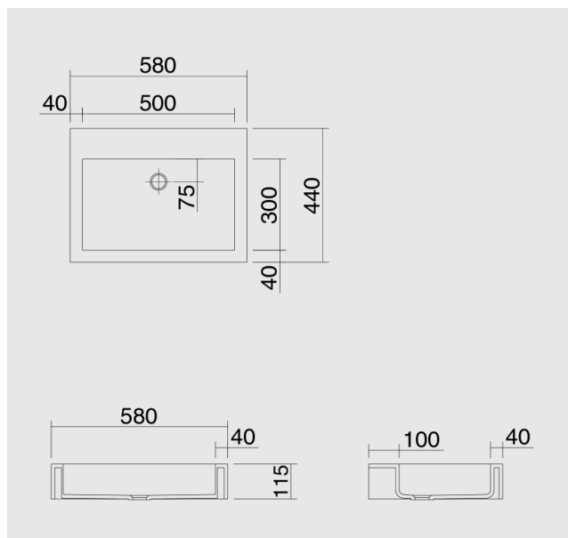
FONTANA ASP-58
