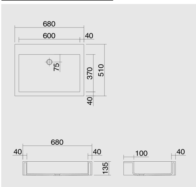
FONTANA ASP-68
